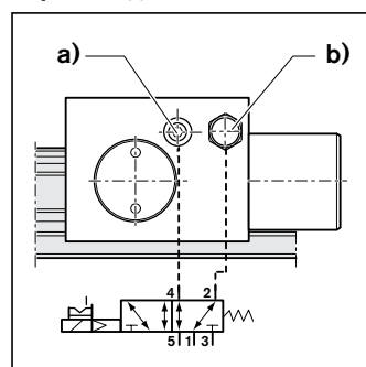
Схема 2) подвода воздуха через вход PLUS
