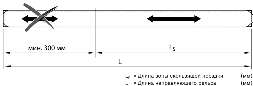
Защитная лента с зоной скользящей посадки
