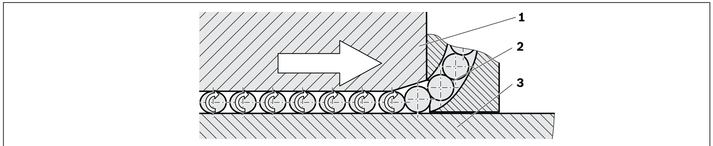
1) Шариковая каретка 2) Шарик 3) Направляющий рельс
