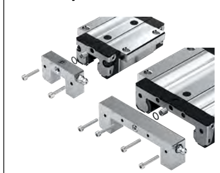
Шприц-масленки
